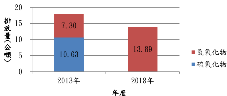
2013年與2018年硫氧化物與氮氧化物總排放量差異
