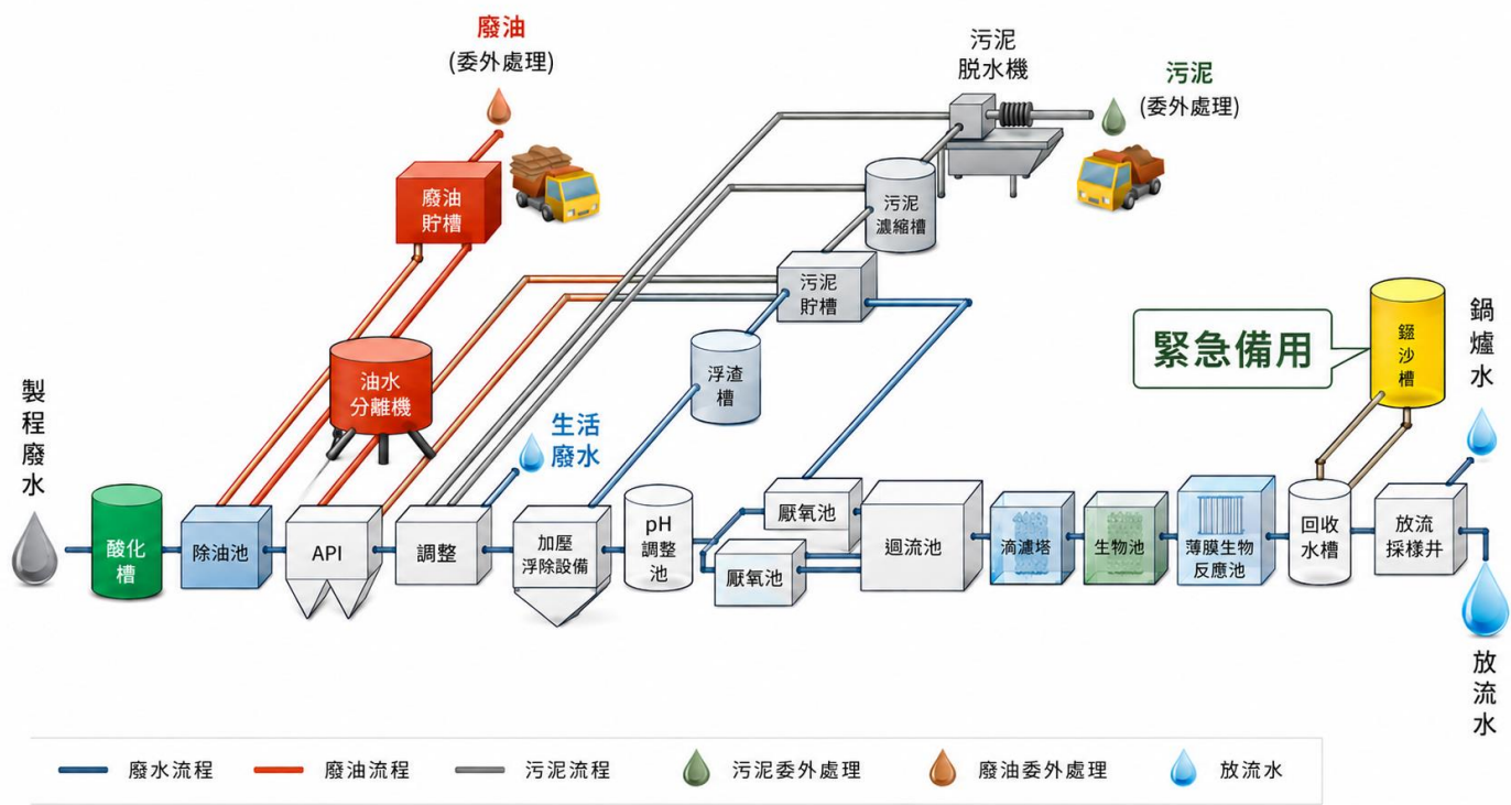
台中港廠廢水處理流程圖
